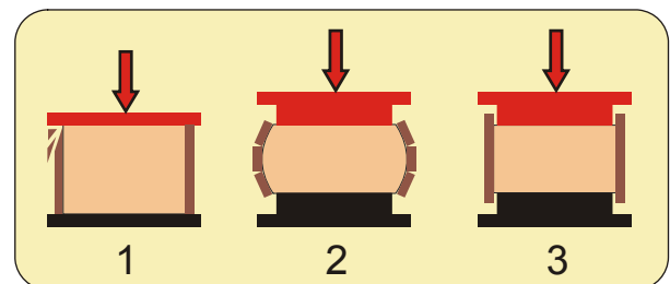
Abbildung 5.13: Beobachtete Versagensarten von verputzten HD-Bällen
