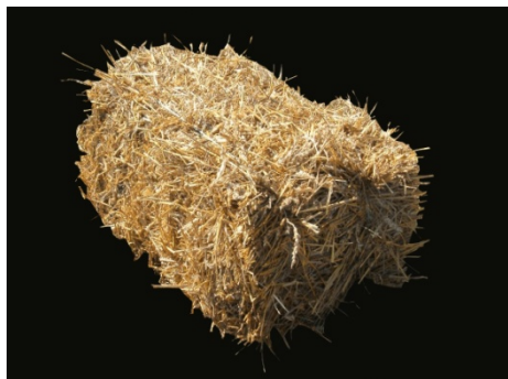
Abbildung 4.5 Lockere Ballen mit unscharfen Kanten müssen aufwändig vorbereitet werden, um als Baustrohballen eingesetzt werden zu können. Notwendige Arbeiten sind das Trimmen (begradigen der Ballenenden), das Rasieren (entfernen überstehender Halme vor dem Verputzen) und evtl. ein Nachverdichten. Ballen unter einer Rohdichte von 110 \text{ kg/m}^2 sollten für das lasttragende Bauen nicht verwendet werden.
