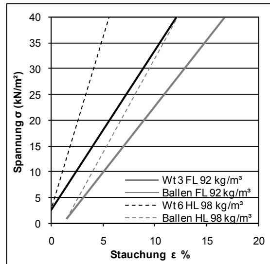
Abbildung 5.35: Vergleich der Elastizitätsmodule und Nullpunktverschiebungen bei unverputzten Einzelballen und Wänden aus Weizenstroh
