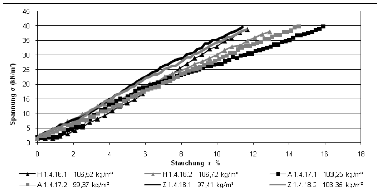
Abbildung 2.27: Spannungs-Stauchungsdiagramm unverputzter flach liegender halbiertes Weizenballen mit seitlicher Einspannung
