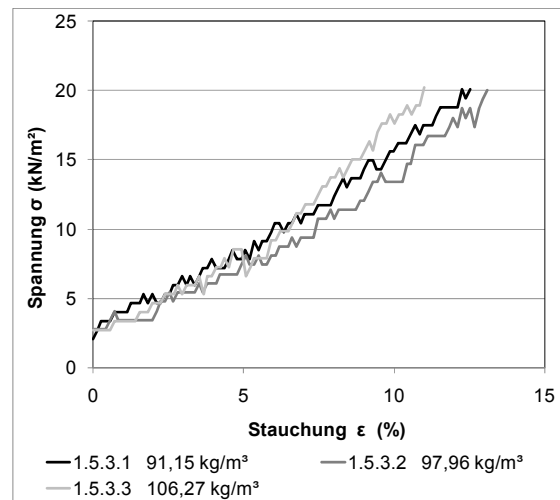
Abbildung 2.30: Spannungs-Stauchungsdiagramm Weizenballen stehend, unverputzt ohne seitliche Einspannung
