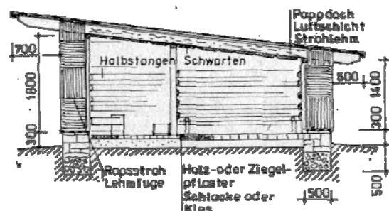
Abbildung 1.3: Tierstall in der ehemaligen DDR (Gratz 1988: 131)
