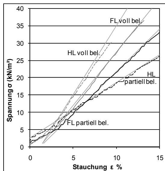
Abbildung 5.11: Vergleich der Elastizitätsmodule und Spannungs-Stauchungs-Kennlinien voll und partiell belasteter flach und hochkant liegender HD-Weizenballen mit seitlicher Einspannung
