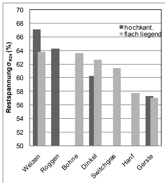
Abbildung 5.24: Vergleich der Restspannung nach 24 Stunden bei eingespannten, nicht verputzten flach- und hochkant liegenden HD-Ballen verschiedener Stroharten im Kombitest bei einer Startspannung von 40 kN/m 2
