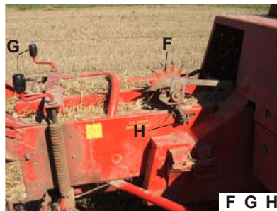
Abbildung 4.4: Zur Funktionsweise von HD-Ballenpressen (Zeichnung: Welger 8: 3, eigene Fotos, Beschriftung, Darstellung)
