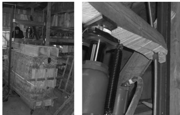
Abbildung 2.29: Großballen 1.6.1.1 während des Tests und Beschädigung am Hauptjoch
