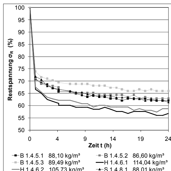
Abbildung 5.3: Relaxationsdiagramm flach liegender unverputzter HD-Gersten- und Dinkelballen mit seitlicher Einspannung im Kombitest ausgehend von einer Startspannung von 40 kN/m 2
