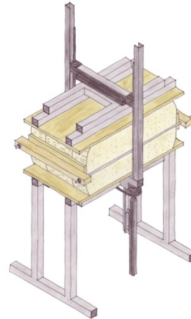
Abbildung 4.2: HD-Kombiprüfstand
