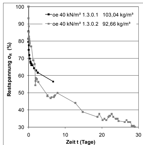
Abbildung 5.6: Relaxationsdiagramm flach liegender unverputzter HD-Weizenballen ohne seitliche Einspannung im Langzeittest \sigma_s = 40 \text{ kN/m}^2
