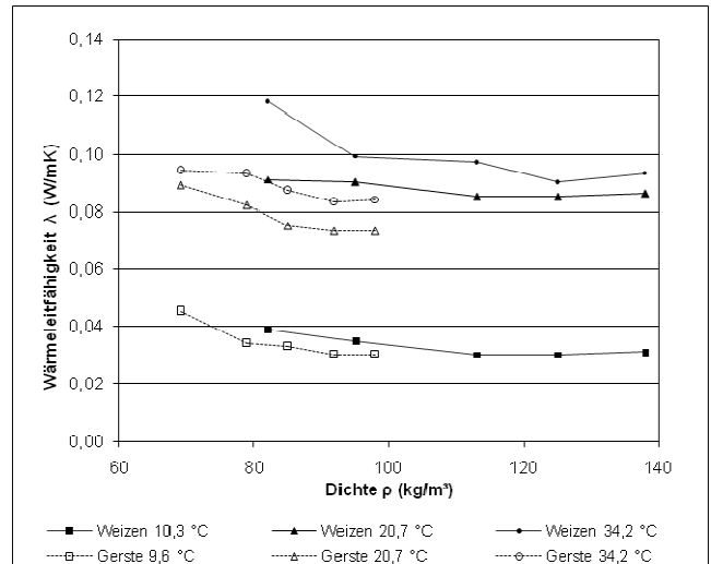
Abbildung 6.1: Wärmeleitfähigkeit von Weizen- und Gerstenstroh in Abhängigkeit von der Dichte (Daten vgl. Ashour 2003: 234, 242)
