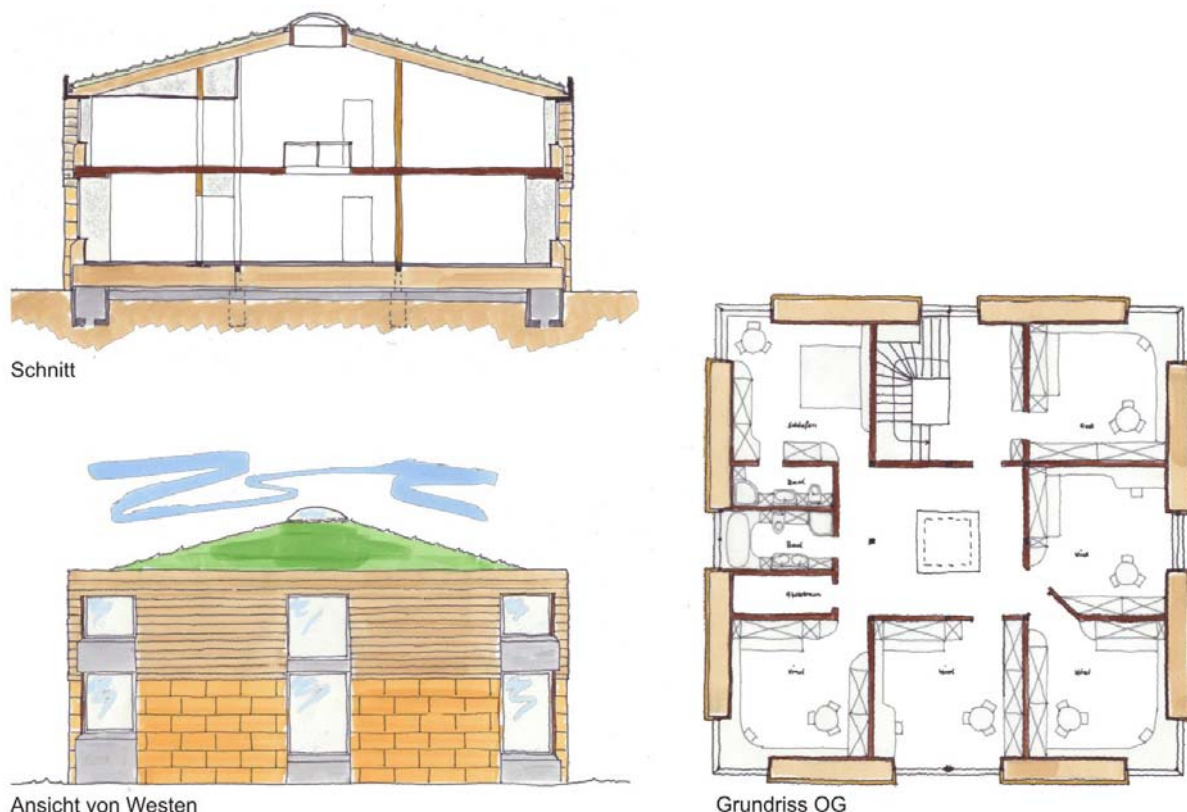
Abbildung 6.3: Skizzen zu dem zweigeschossigen Hybridgebäude (2)
