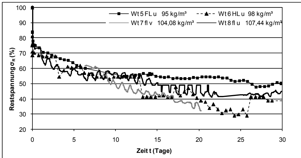
Abbildung 5.33: Relaxationsverhalten der untersuchten Wände bei einer Startspannung von 40 \text{ kN/m}^2
