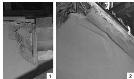
Abbildung 8.8: Putzbrüche infolge von Horizontalspannung (1) und Vertikalspannung (2)
