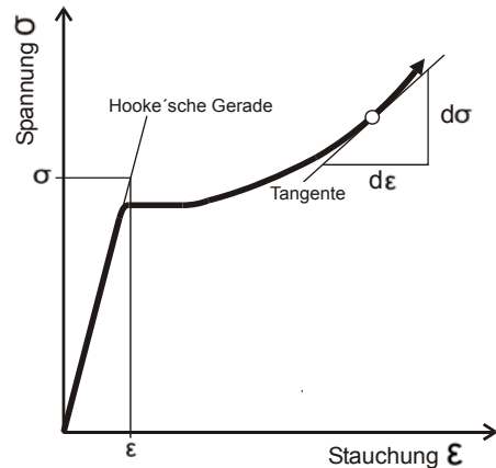
Abbildung 1.6: E-Modul- und Hooke'sche Gerade
