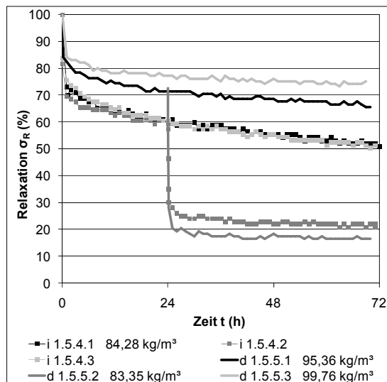
Abbildung 5.13: Relaxationsdiagramm verputzter hochkant liegender HD-Weizenballen mit seitlicher Einspannung ausgehend von einer Startspannung von 40 kN/m 2
